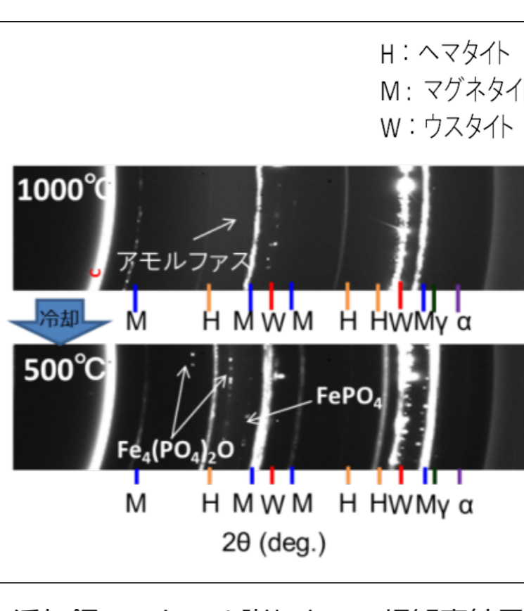
P添加鋼のスケール剥れとその場観察結果
