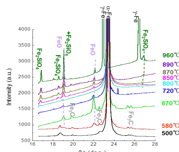
Si添加鋼の初期スケール成長のその場観察
