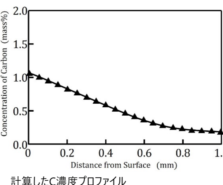
析出物がある場合の浸炭深さの計算例
