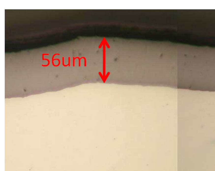
SFCによるTiAlN厚膜形成例
