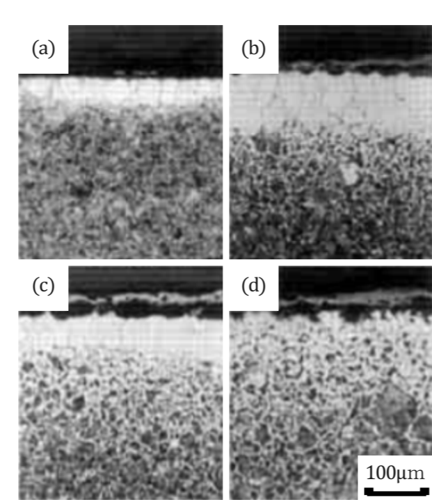
フェライト脱炭を起こした鋼材の断面図
