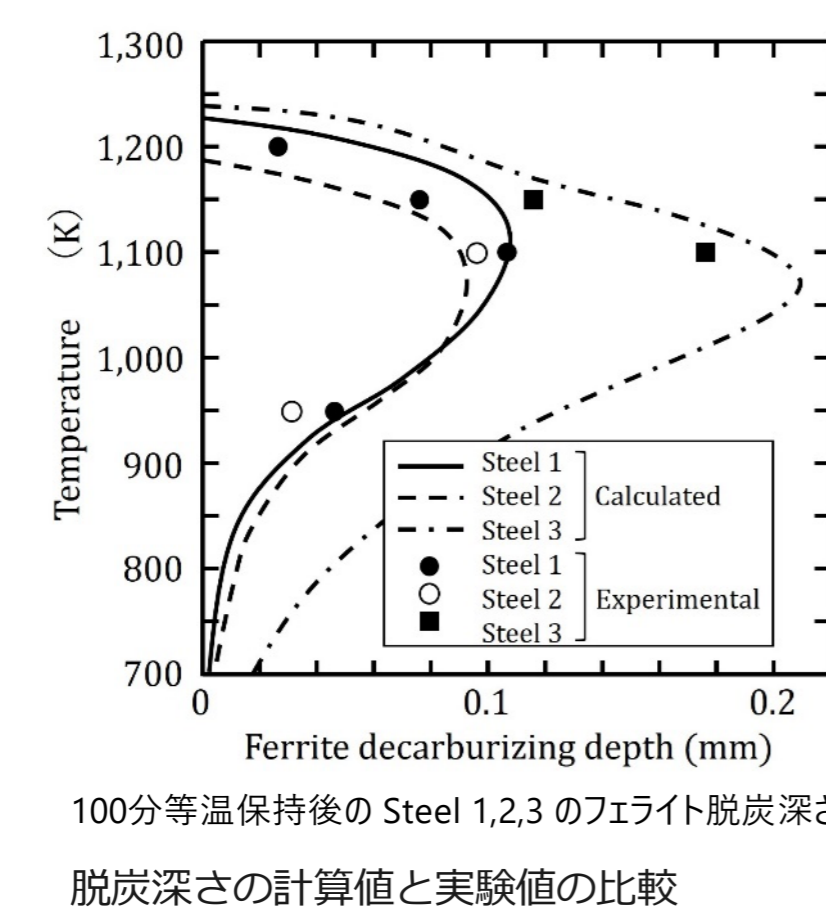
脱炭深さの計算値と実験値の比較
