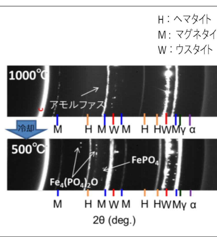
P添加鋼のスケール膨れとその場観察結果
