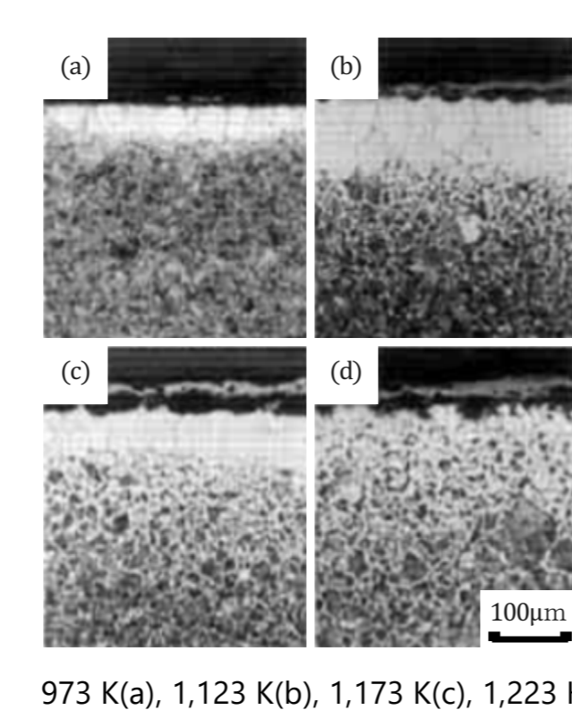
フェライト脱炭を起こした鋼材の断面図
