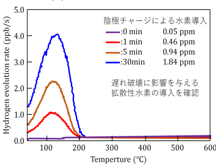
TDSによる陰極チャージで水素を導入した材料の水素放出曲線
