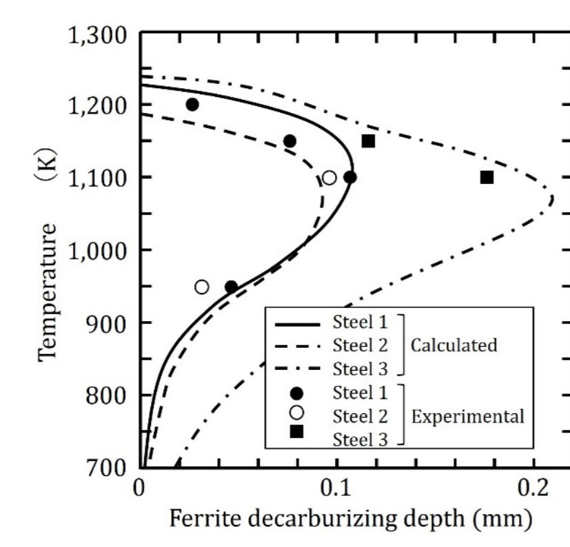
脱炭深さの計算値と実験値の比較
