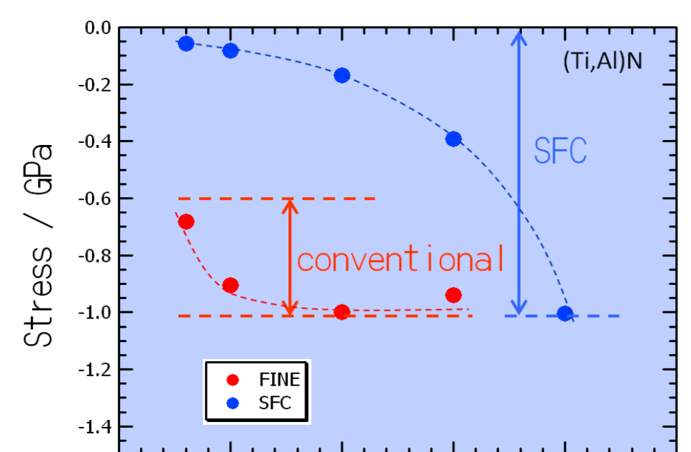
SFCは従来蒸発源に比べ、印加電圧を制御することにより、幅広い範囲で応力制御が可能
