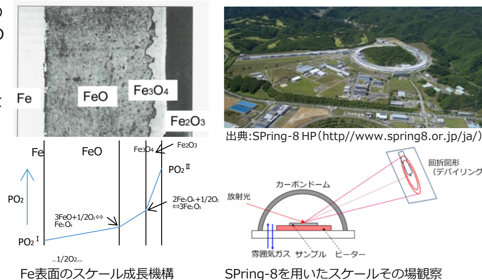
SPring-8を用いたスケールその場観察
