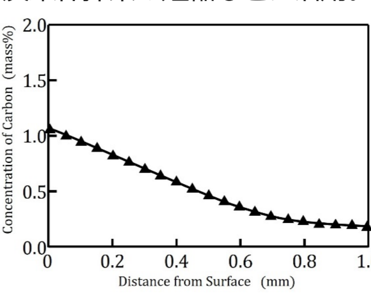
析出物がある場合の浸炭深さの計算例
