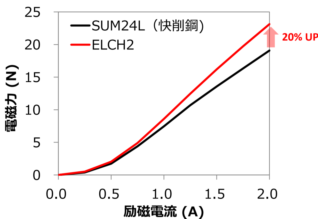
自動車用電磁弁における電磁力比較（解析結果） ※ELCH2：当社純鉄軟磁性材料
