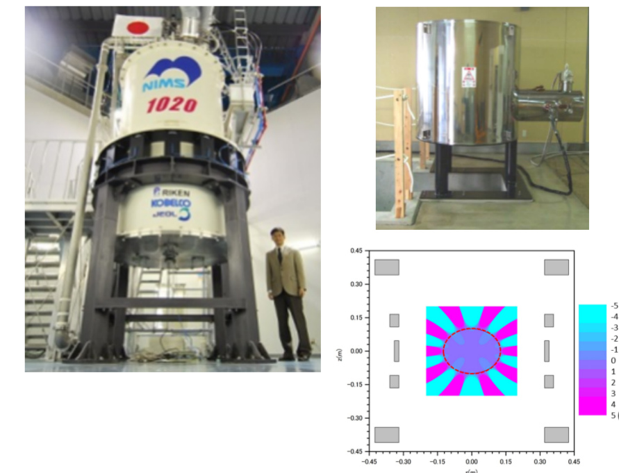
世界最高磁場*の1.02 GHz (24.0T)NMR マグネット(左上) ※2015/4/17時点 頭部用超電導3T-MRIマグネット(右上) MRIマグネットの均一磁場設計(右下)
